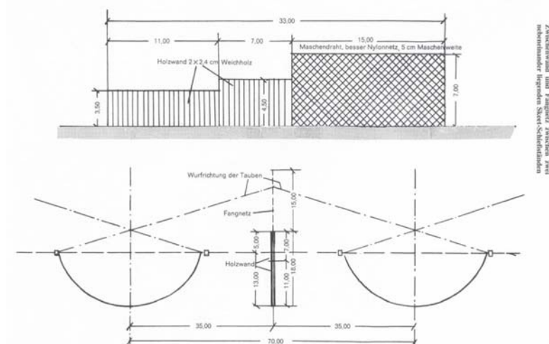
Abbildung 9.6.2.3 Trennwand zwischen zwei nebeneinander liegenden Skeet-Ständen
