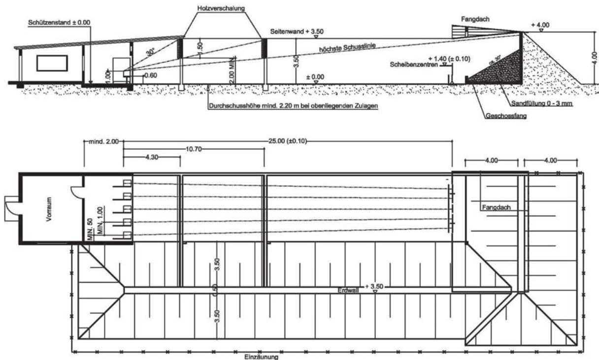
Abbildung 4.8.1 25-m-Schießstand
