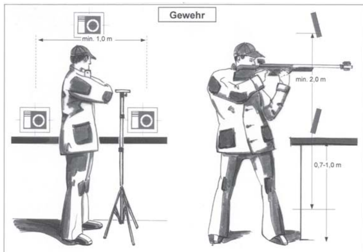
Abbildung 3.1.1 Abmessungen am Schützenstand für DL-Waffen
