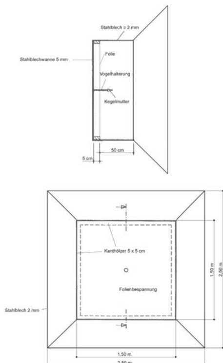
Abbildung 7.9.6 Geschossfang für Flinten mit Schrot auf Vogelschießständen
